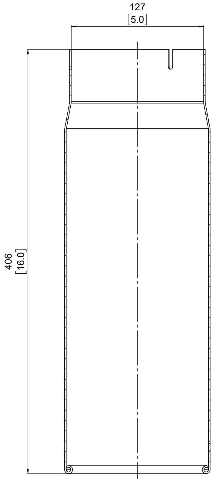
SECTION A-A
