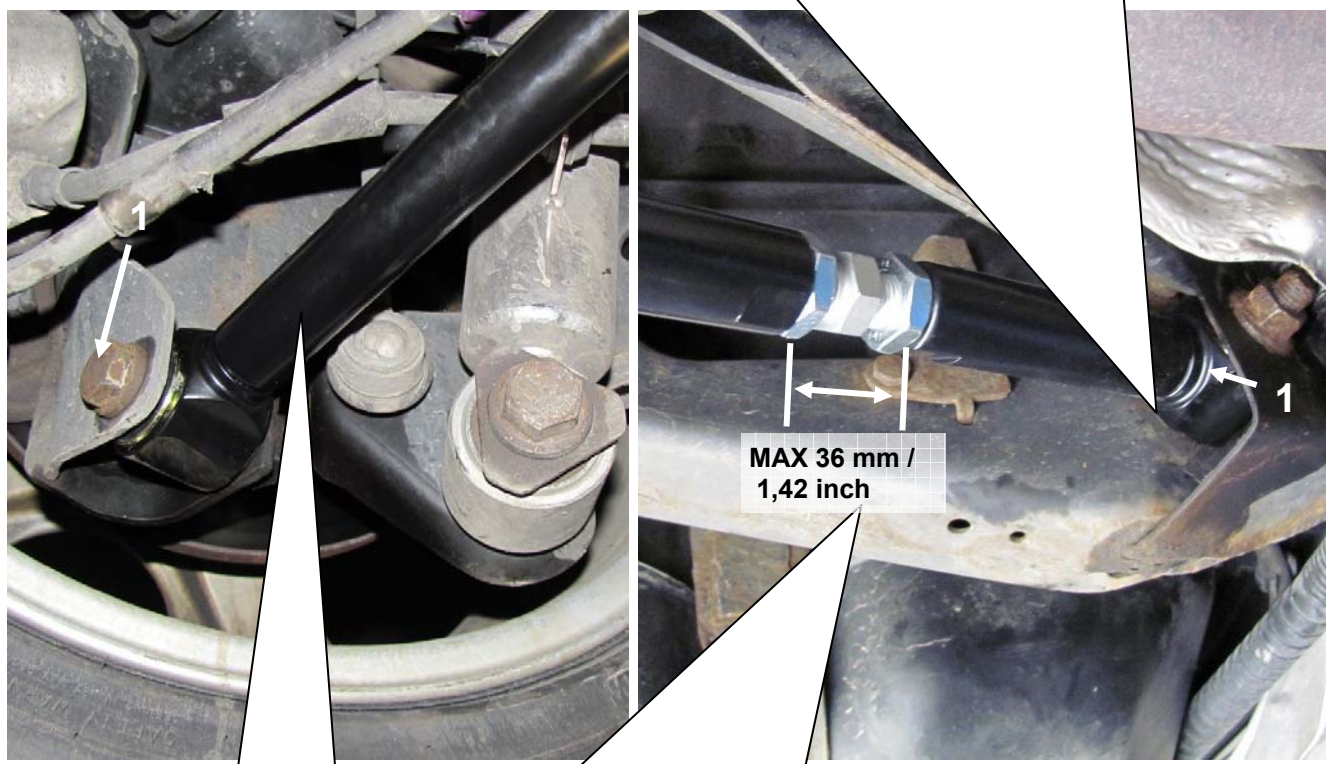
Eingebauter KW Querlenker.
